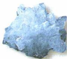
Крупная градина и её строение
