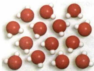
Жидкая вода
