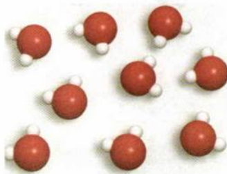
Водяной пар
