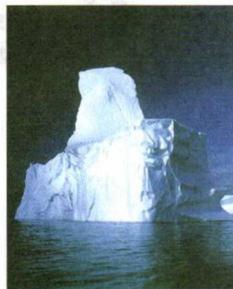
Изменение состояния воды
