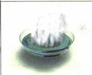
Выделяется тепло
