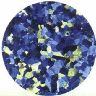
кристаллы железа
