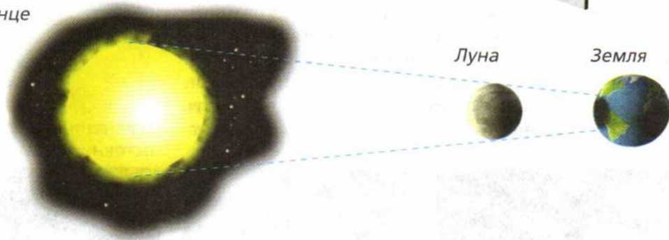
Солнце
