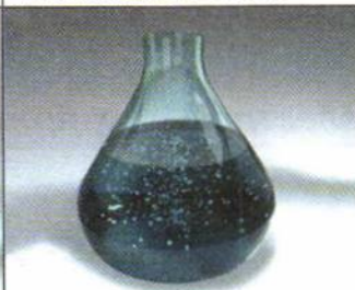
Выделяется газ
